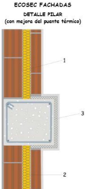
Fig. 3. Detalle de encuentro con pilar
