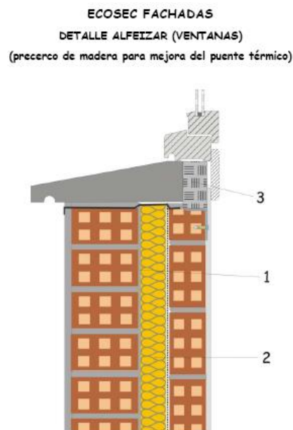
Fig. 6. Detalle de encuentro con ventana
