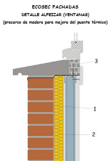
Fig. 12. Detalle de encuentro con ventana
