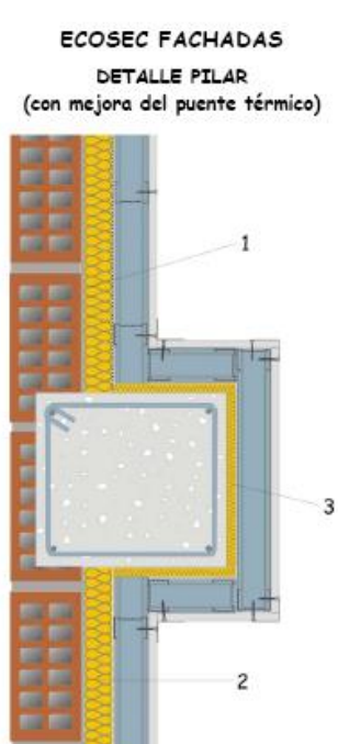
Fig. 10. Detalle de encuentro con pilar
