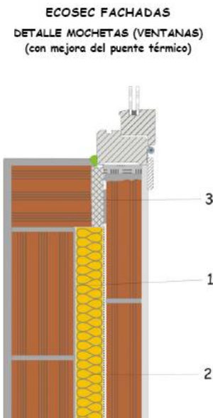
Fig. 5. Detalle de encuentro con ventana
